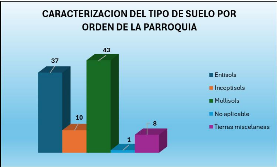
Gráfico 3 Caracterización de suelos, número de hectáreas y porcentaje
