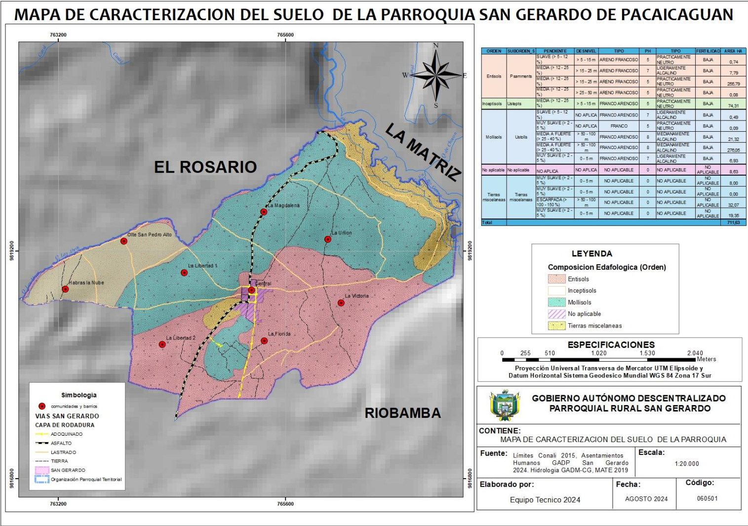
Mapa 6 Mapa de Caracterización del Suelo de la Parroquia San Gerardo de Pacaicaguán
