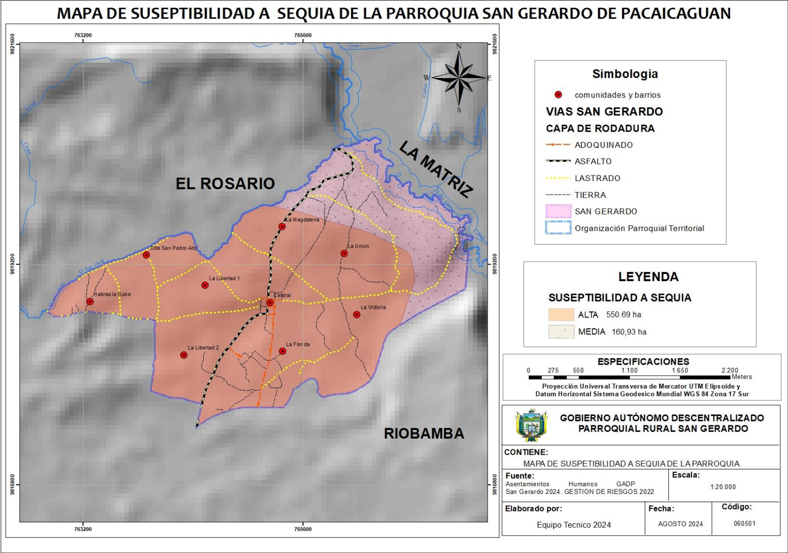
Mapa 15 Susceptibilidad a sequia de la Parroquia San Gerardo de Pacaicaguán
