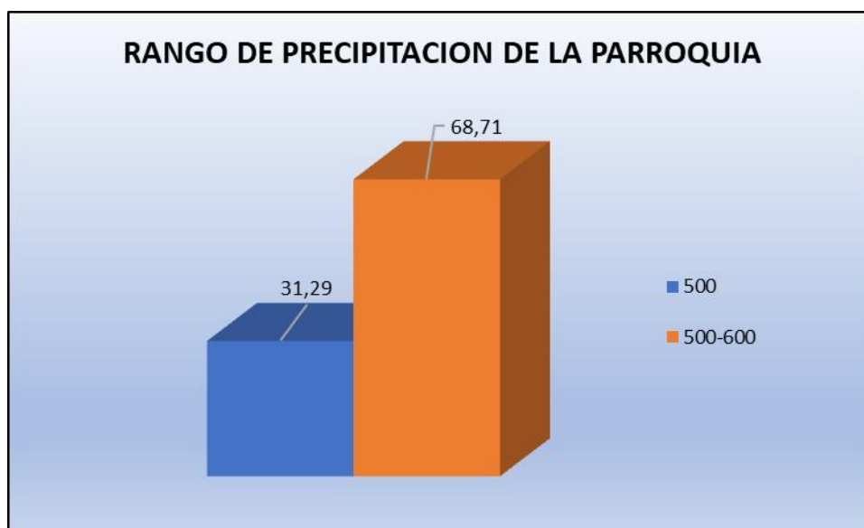
Gráfico 10 Rango de Precipitación anual acumulada
