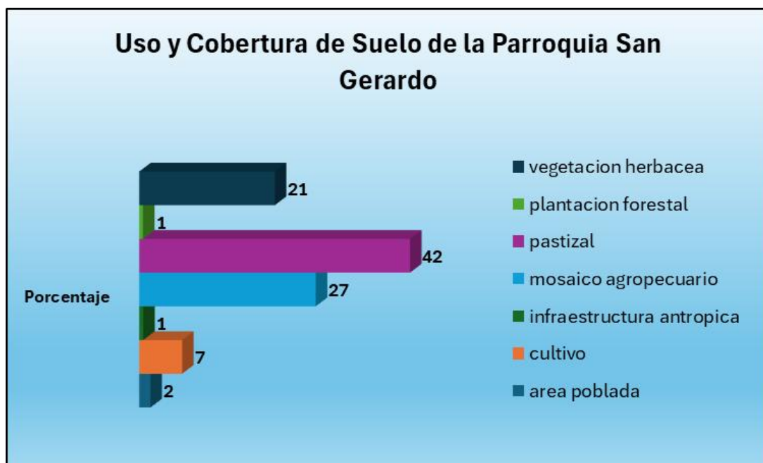
Gráfico 4 Cobertura del suelo.
