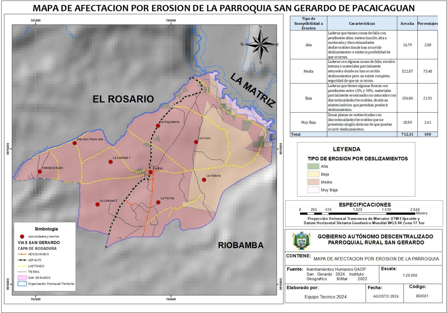
Mapa 18 Zonas de erosión por deslizamientos de la Parroquia
