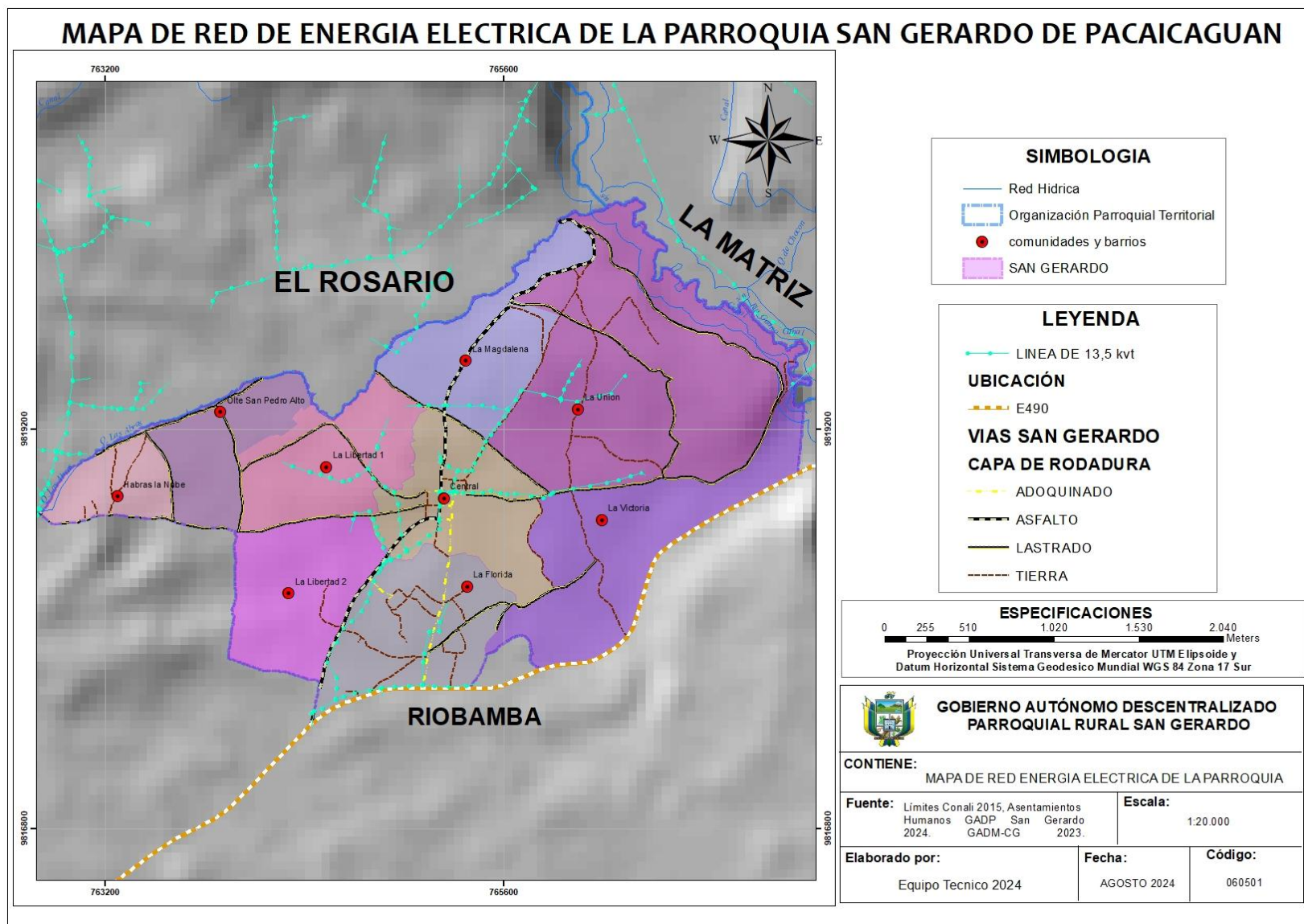
Mapa 28 Red de Energía Eléctrica de la Parroquia San Gerardo de Pacaicaguán
