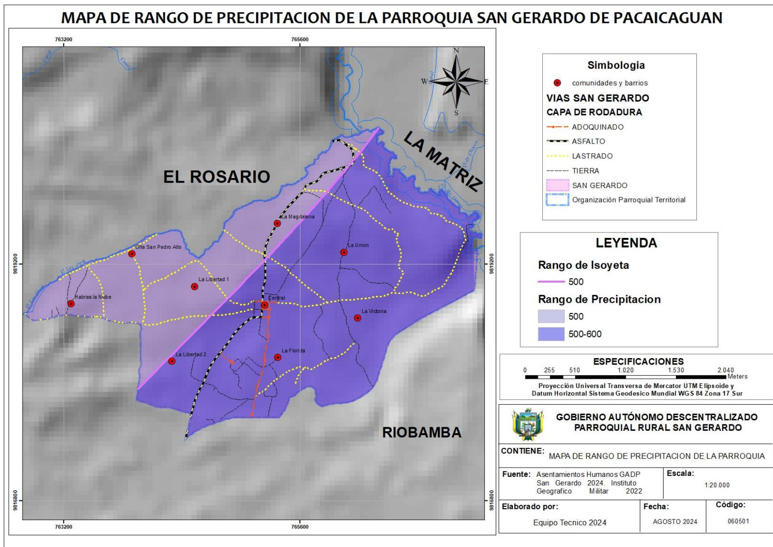
Mapa 17 Rango precipitación de la Parroquia San Gerardo de Pacaicaguán
