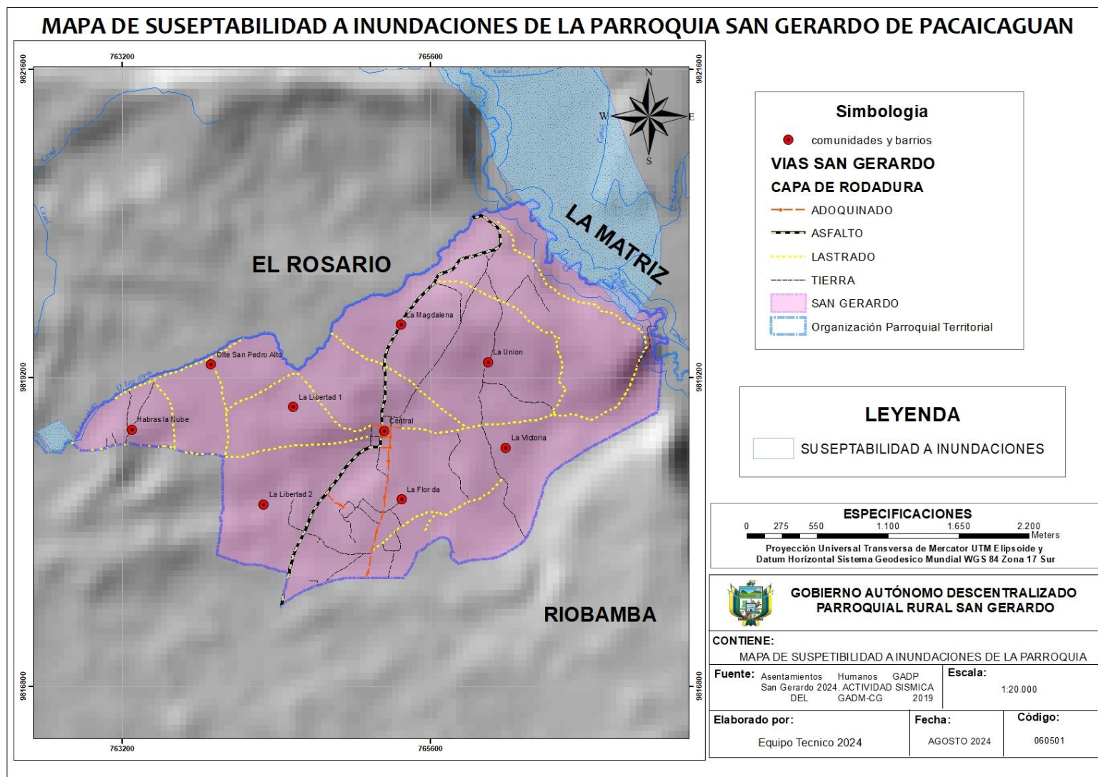
Mapa 13 Susceptibilidad a inundaciones de la Parroquia San Gerardo de Pacaicaguán
