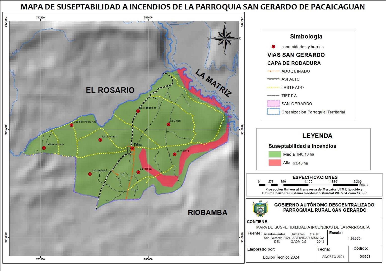
Mapa 14 Susceptibilidad a incendios de la Parroquia San Gerardo de Pacaicaguán
