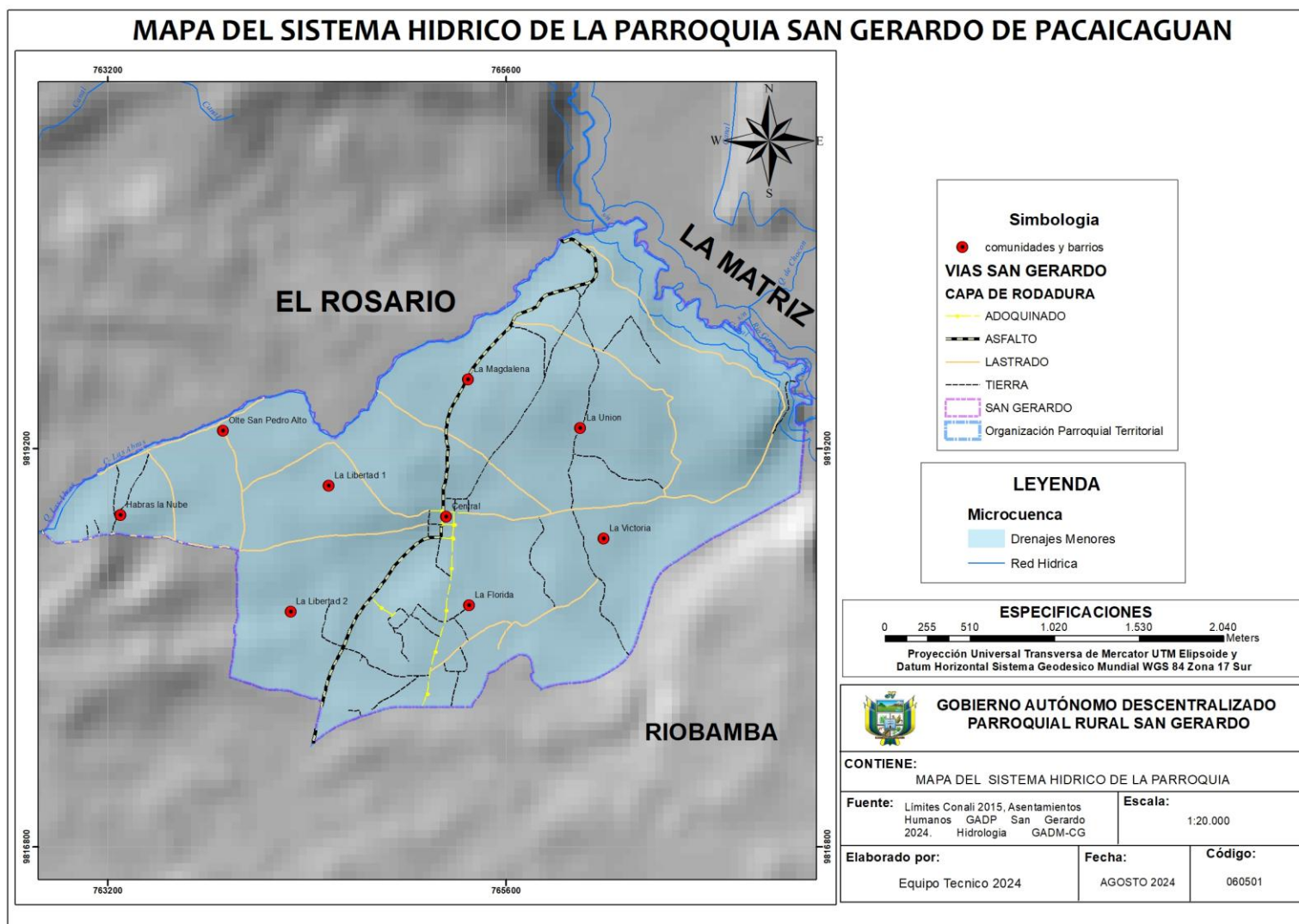
Mapa 3 Sistema hídrico de la Parroquia San Gerardo de Pacaicaguán
