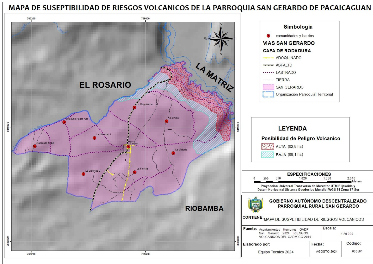
Mapa 10 Riesgo volcánico de la Parroquia San Gerardo de Pacaicaguán
