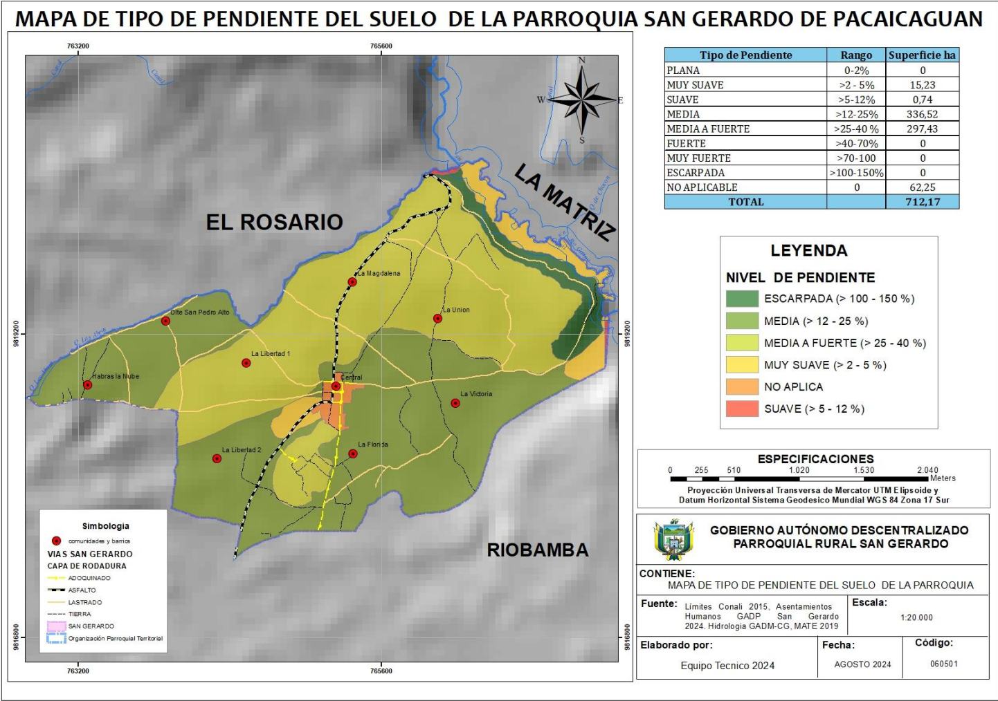
Mapa 36 Pendientes del suelo de la Parroquia San Gerardo de Pacaicaguán
