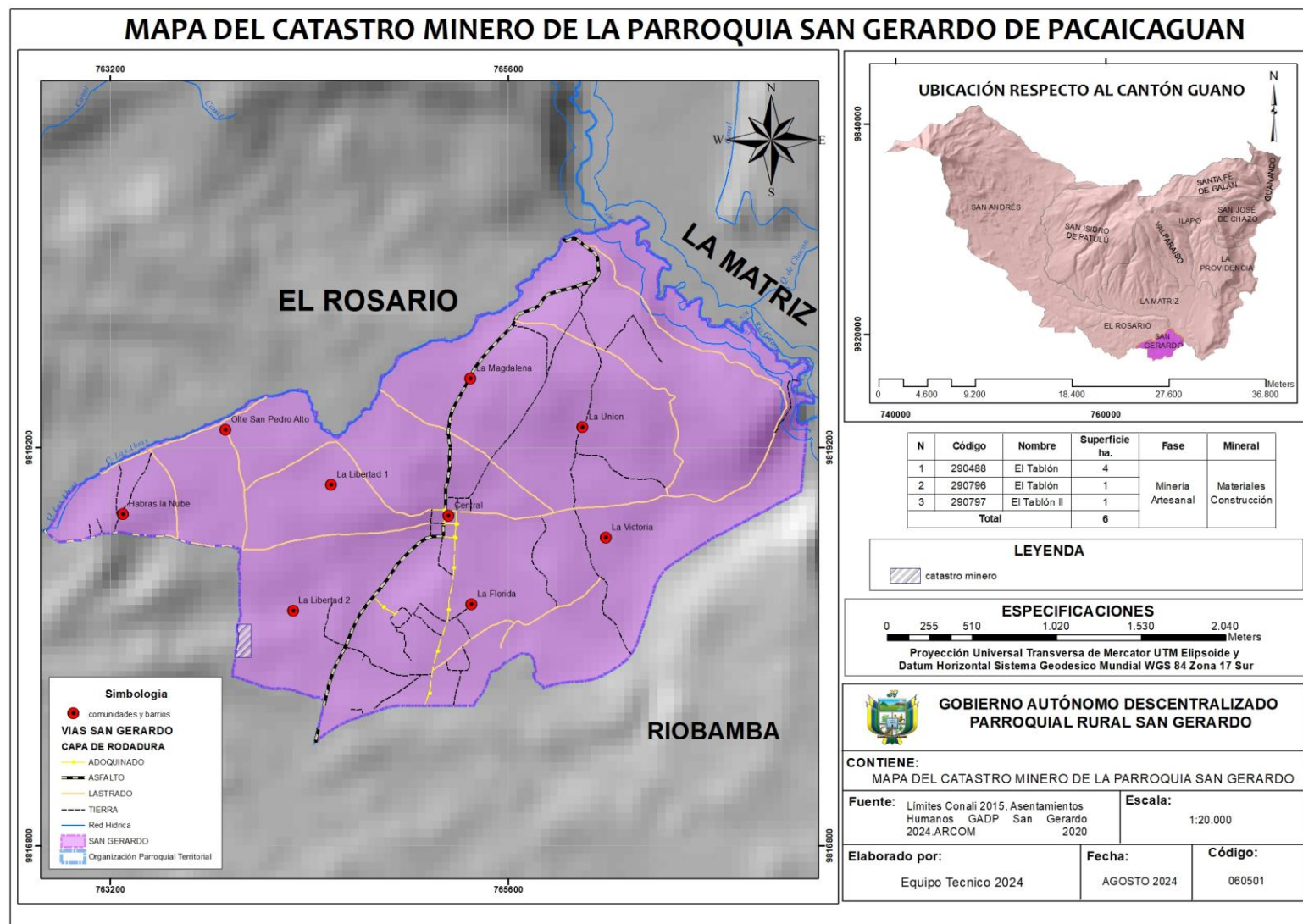
Mapa 2 Concesiones mineras de la Parroquia San Gerardo de Pacaicaguán
