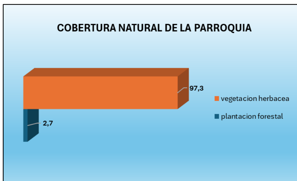
Gráfico 2 Cobertura vegetal existentes en la Parroquia San Gerardo de Pacaicaguán
