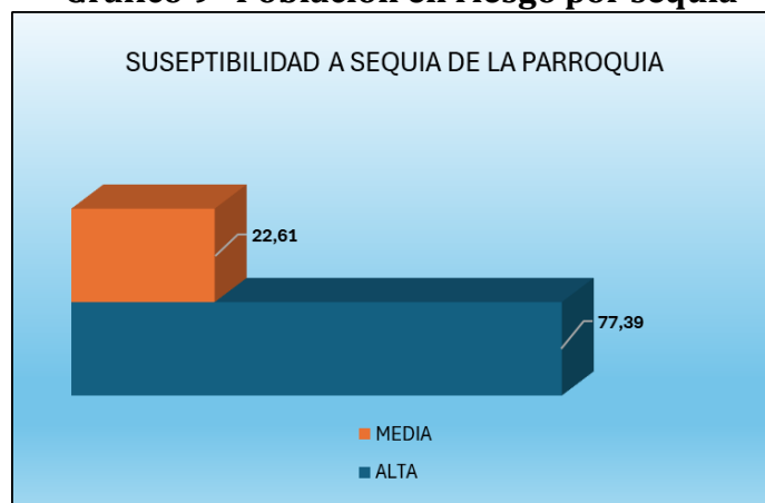
Gráfico 9 Población en riesgo por sequia
